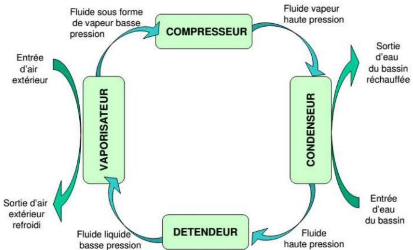
Figure 2. Cycle du fluide frigorigène dans la PAC.
